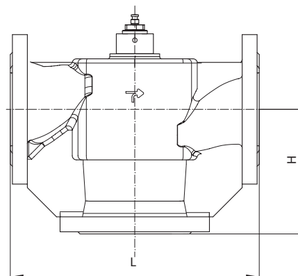
VL 3 (DN 100)
