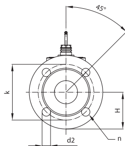
VL2 (DN 15–80)
