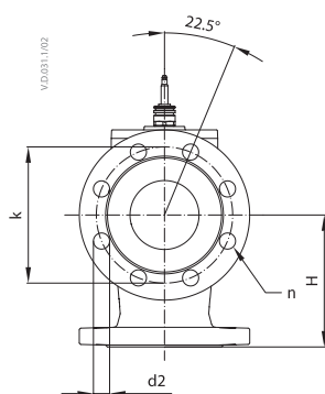
VF 3 DN 80
