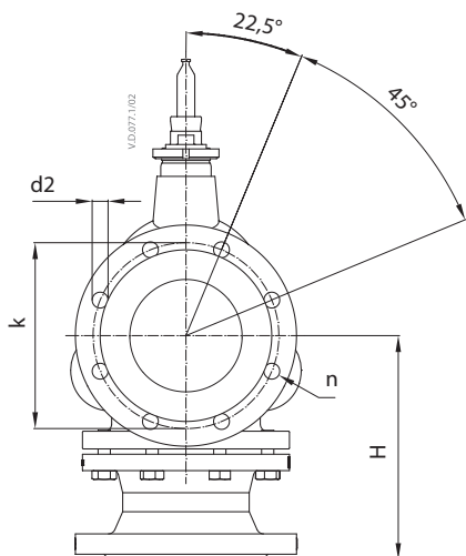
VF 3 DN 125-150
