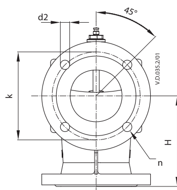
VL 3 (DN 100)
