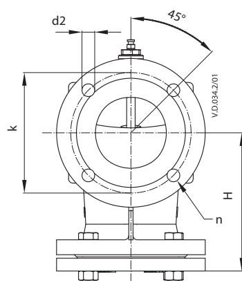
VL 2 (DN 100)
