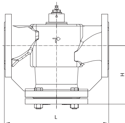
VL 2 (DN 100)
