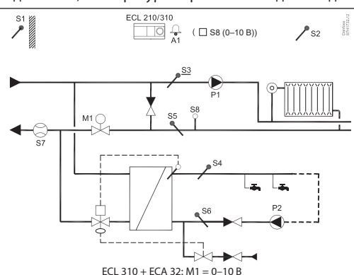
Приложение A230.4d. Зависимая система отопления. Опциональная функция мониторинга давления, температуры горячей и холодной воды
