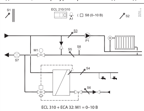
Приложение A230.4c. Зависимая система отопления. Опциональная функция мониторинга давления, температуры горячей и холодной воды
