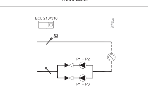
Приложение A230.2d. Схема управления работой установки со спаренными циркуляционными насосами
