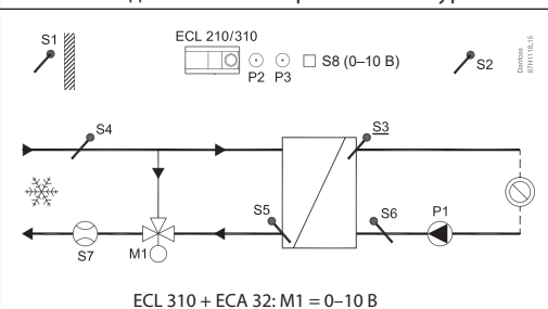
Приложение A230.2c. Система централизованного холодоснабжения с промежуточным теплообменником и постоянным расходом холодоносителя в первичном контуре
