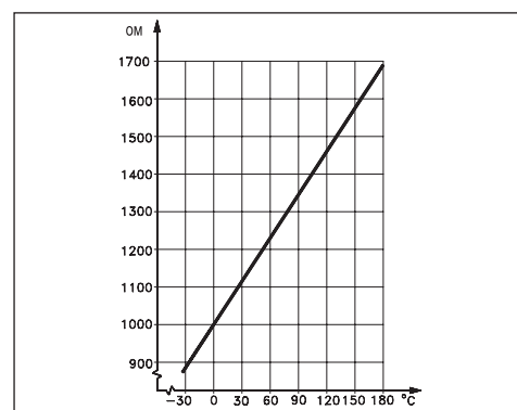
График изменения сопротивления датчика от температуры среды
