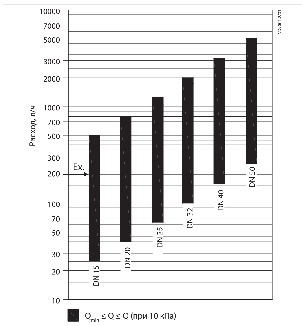
Диаграмма подбора клапана АРТ при \Delta P_{6к} = 10 кПа
