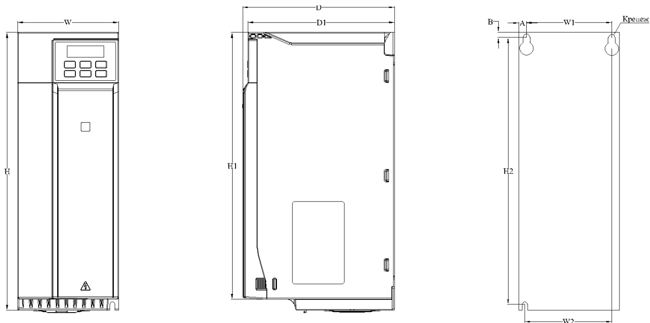
Рис.2-6.3. Чертеж преобразователя частоты типоразмер 3
