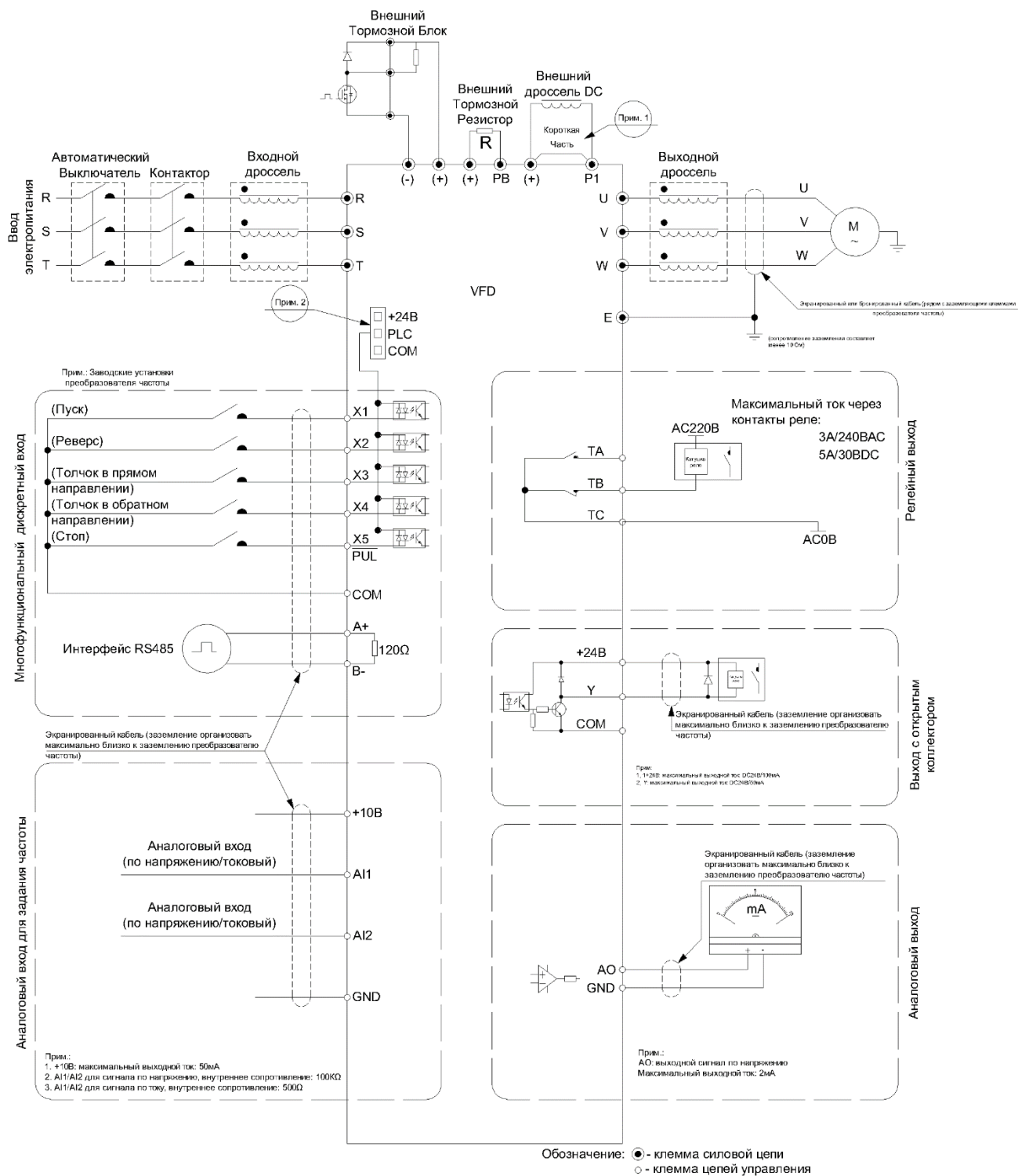
Рис. 3-4. Схема внешних подключений
