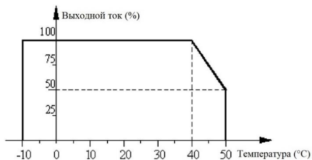
Рис. 2-4. Снижение характеристик преобразователя частоты при превышении допустимой температуры и высоты
