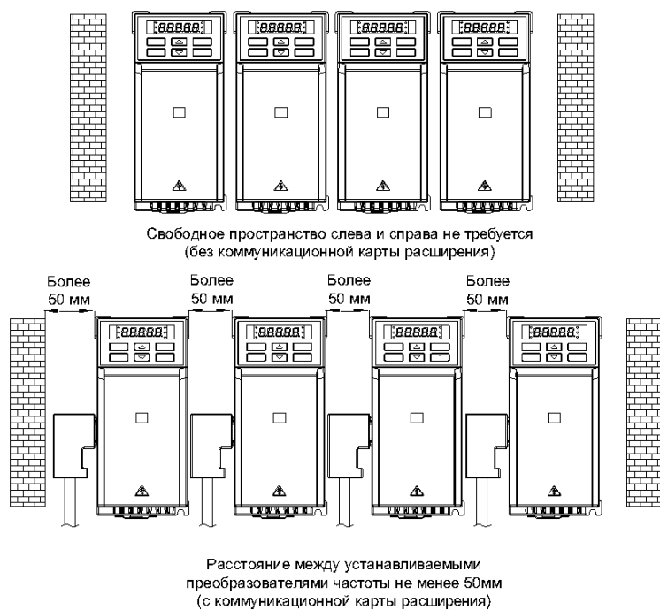
Рис. 2-5. Положение преобразователя частоты и требуемое пространство
