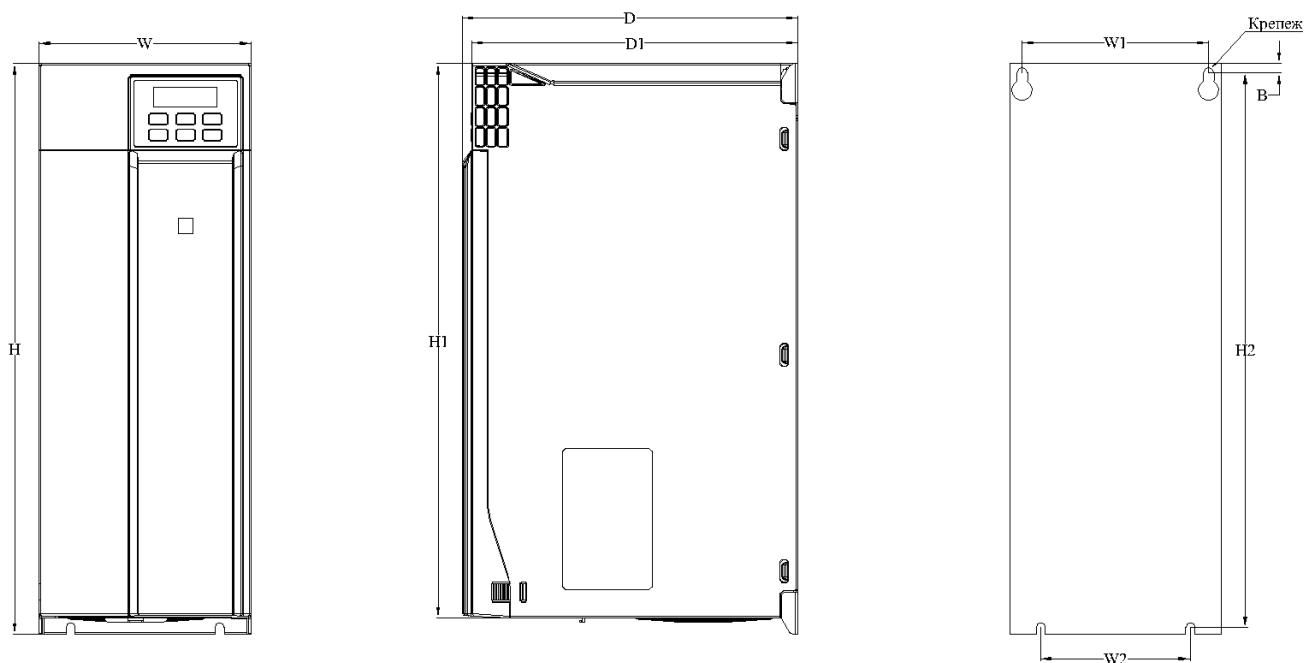
Рис.2-6.4. Чертеж преобразователя частоты типоразмер 4
