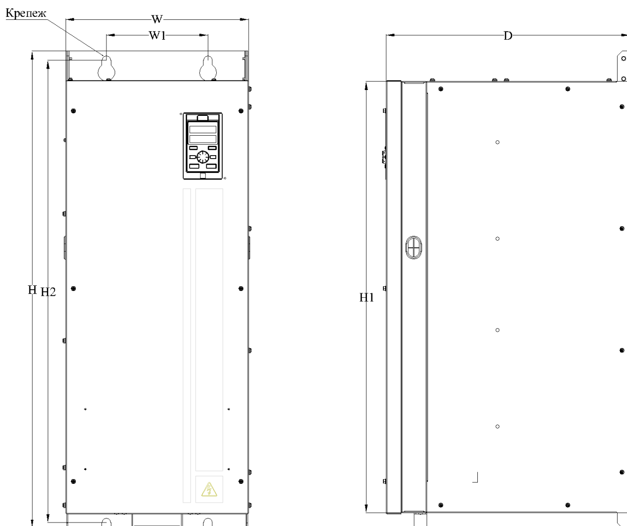
Рис.2-6.8. Чертеж преобразователя частоты типоразмер 8
