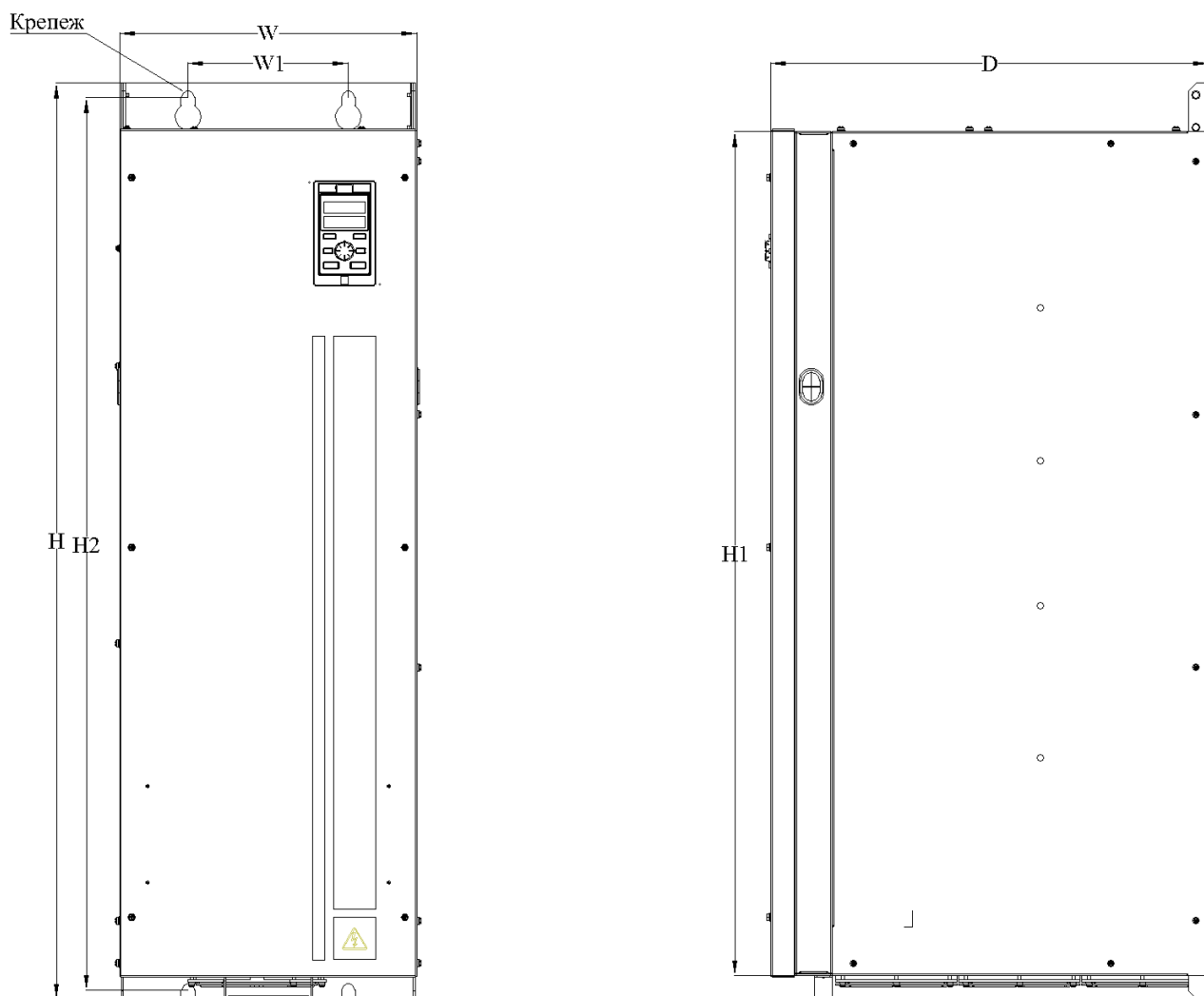
Рис.2-6.9. Чертеж преобразователя частоты типоразмер 9
