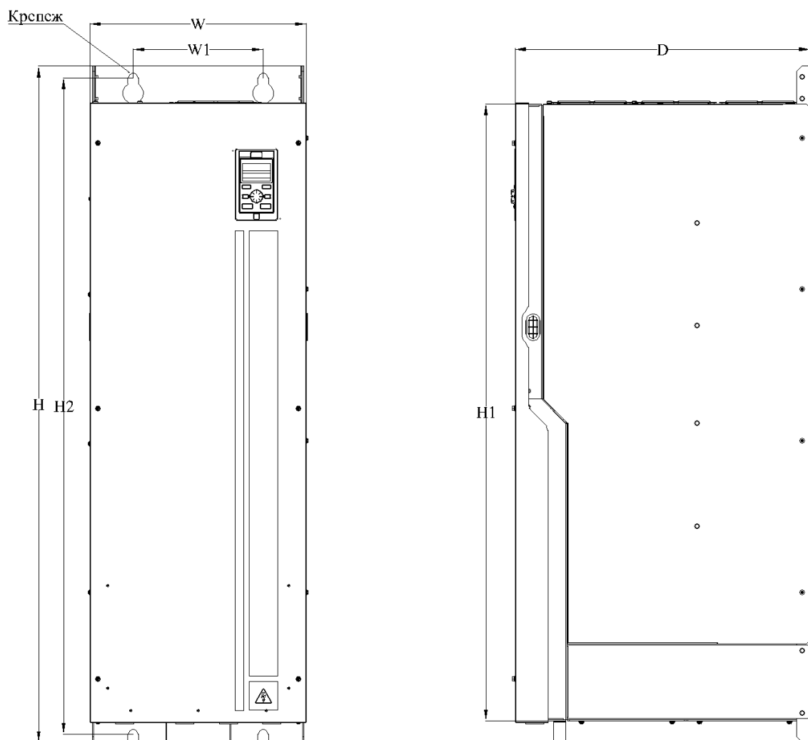
Рис.2-6.10. Чертеж преобразователя частоты типоразмер 10
