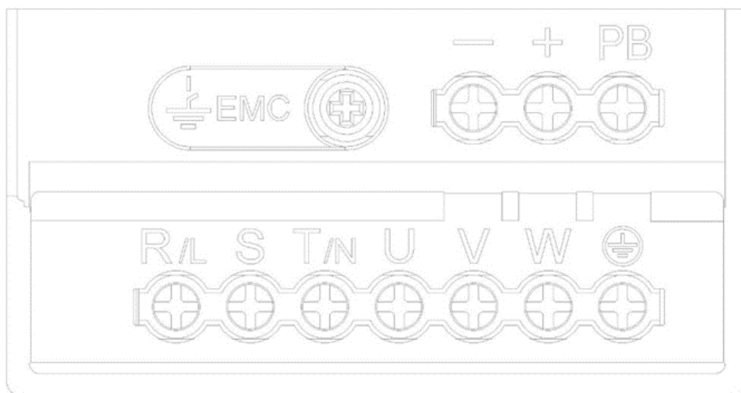
Рис. 3-3.2. Расположение клемм
