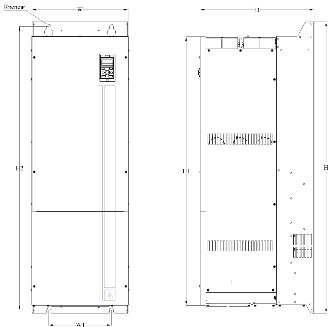
Рис.2-6.11. Чертеж преобразователя частоты типоразмер 11
