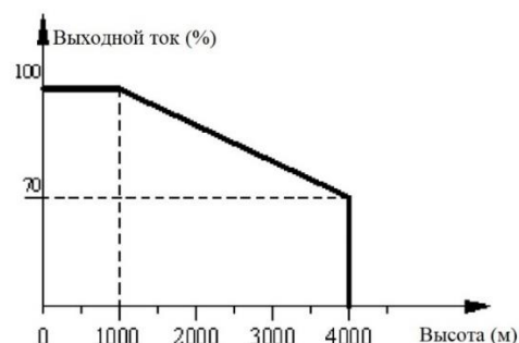
Рис. 2-4. Снижение характеристик преобразователя частоты при превышении допустимой температуры и высоты
