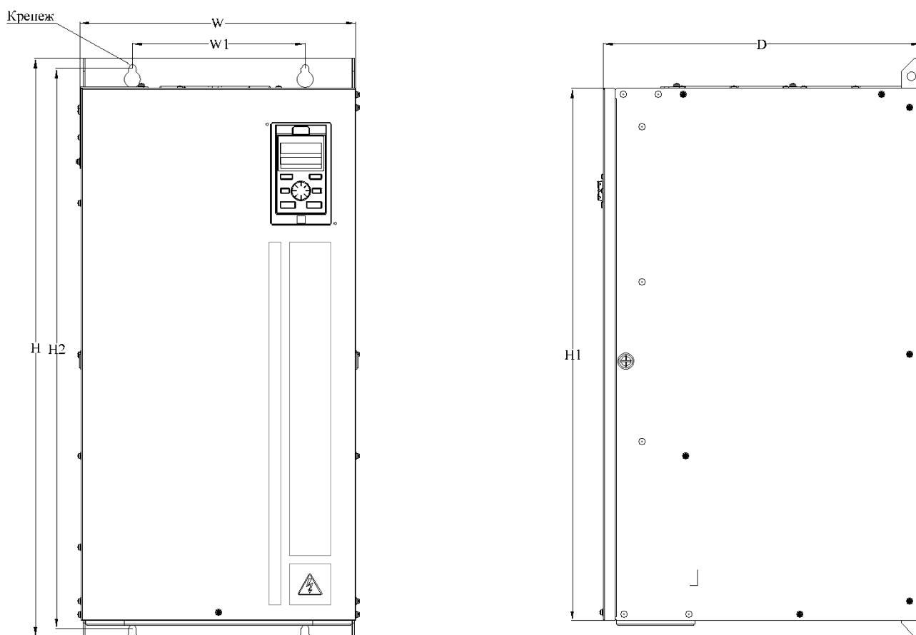
Рис.2-6.7. Чертеж преобразователя частоты типоразмер 7
