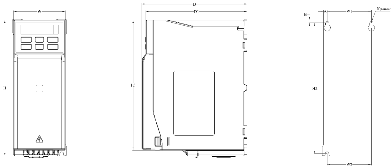
Рис.2-6.1. Чертеж преобразователя частоты типоразмер 1
