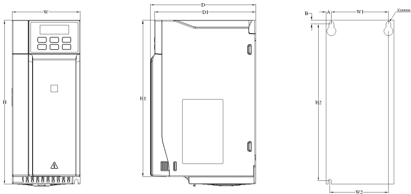
Рис.2-6.2. Чертеж преобразователя частоты типоразмер 2
