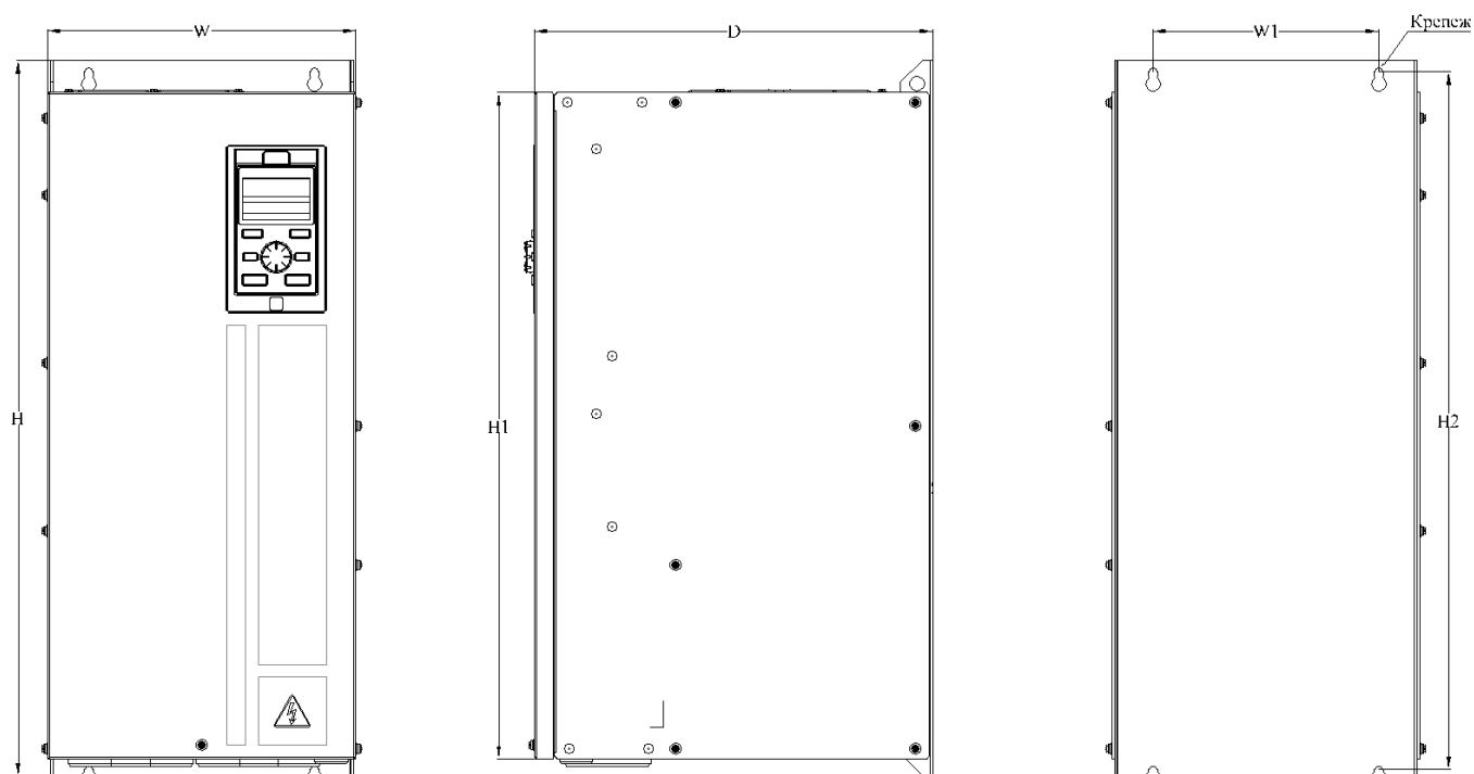
Рис.2-6.6. Чертеж преобразователя частоты типоразмер 6
