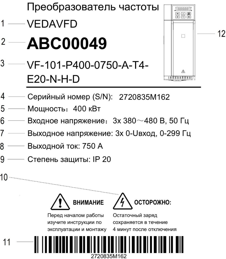
Рис. 1-3. Пример маркировки преобразователя частоты
