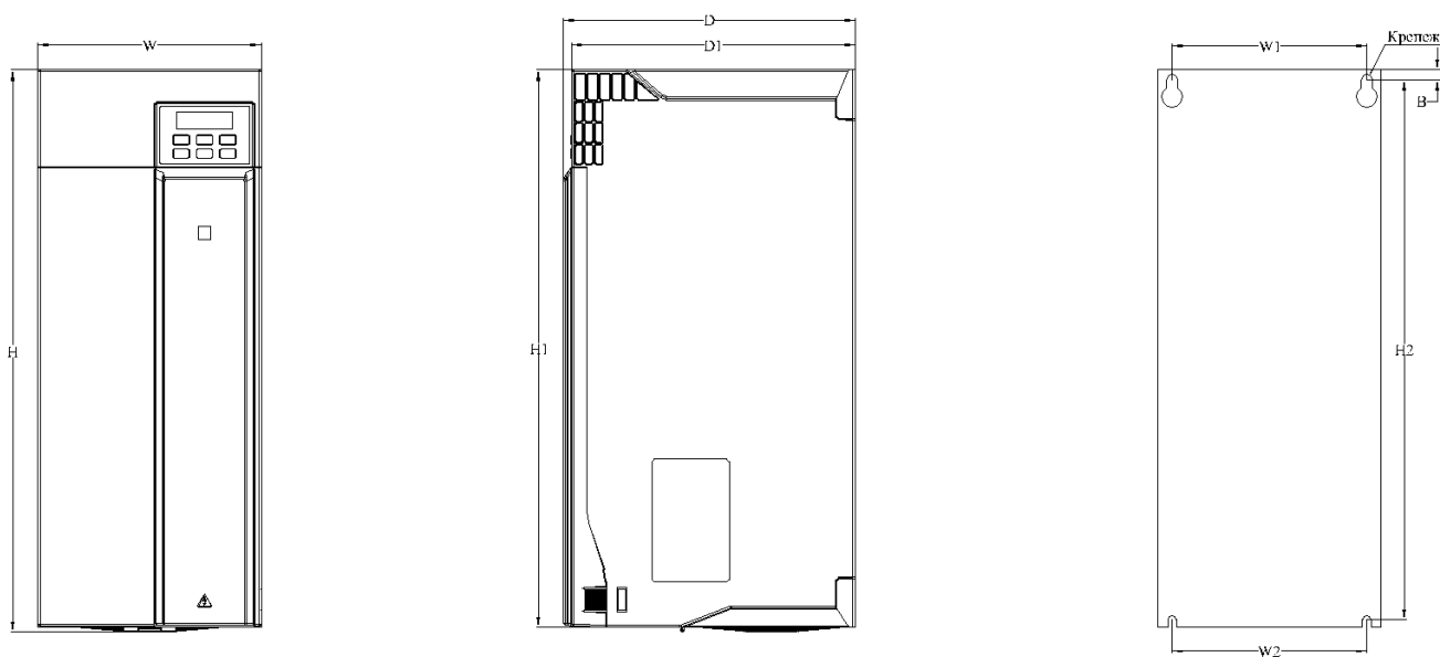
Рис.2-6.5. Чертеж преобразователя частоты типоразмер 5
